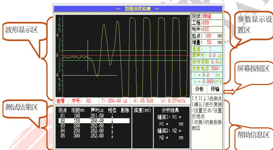
图 4.1 测缝主界面
