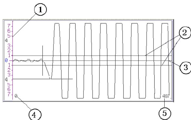
图 5.17 波形显示区
