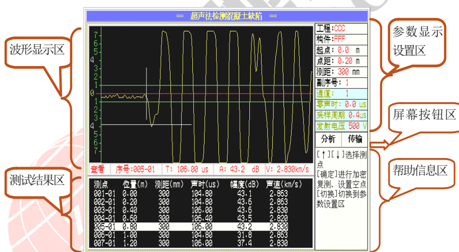
图 3.1 测缺主界面
