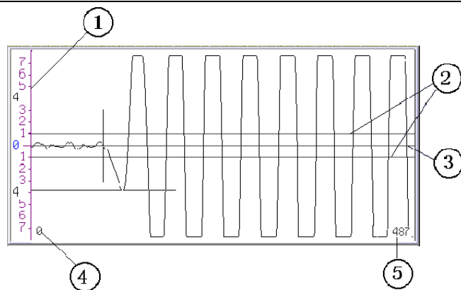
图 4.13 波形显示区
