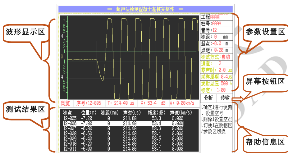
图 2.1 测桩主界面
