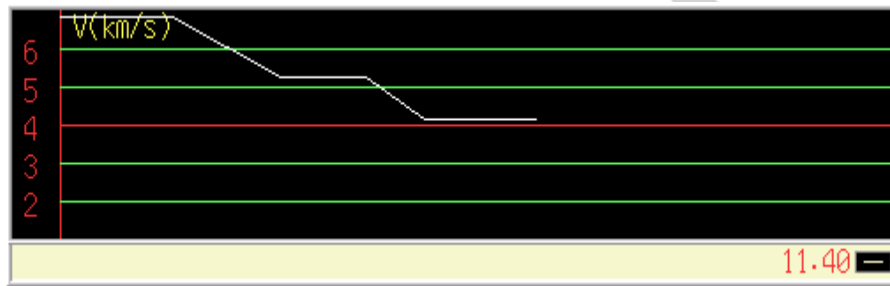
图 6.10 声速曲线
